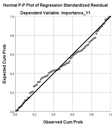
Gambar 2 Uji P-Plot
