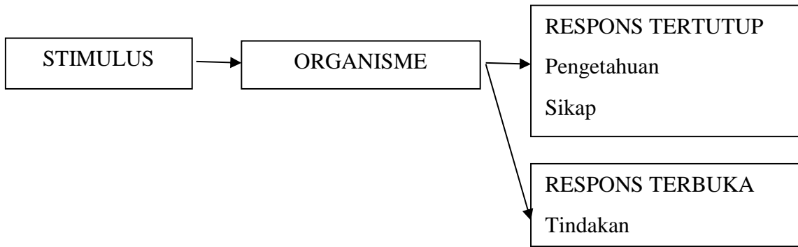
Gambar 2.6 Kerangka Teori
