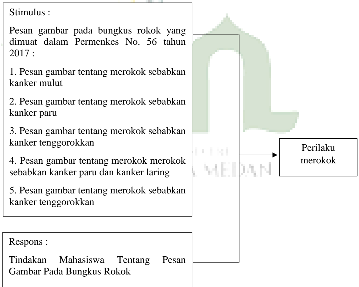
Gambar 2.7 Kerangka Konsep
