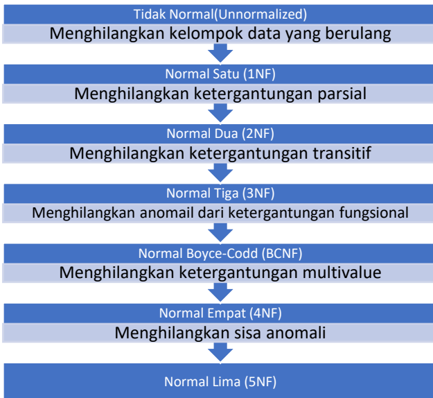
Gambar 6.1. Tahapan Normalisasi
